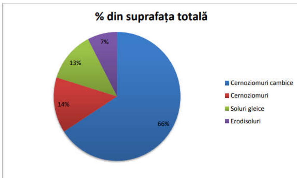
Figura 10: Tipologia solurilor
